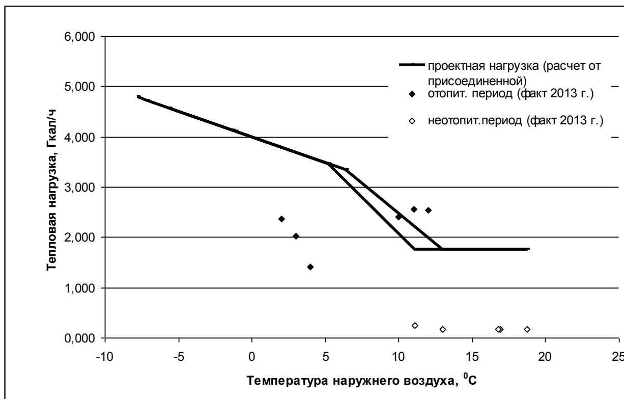
Рисунок 1.30. Зависимость тепловых нагрузок котельной с. Пышлицы ОАО «Водоканал МО» от температуры наружного воздуха
