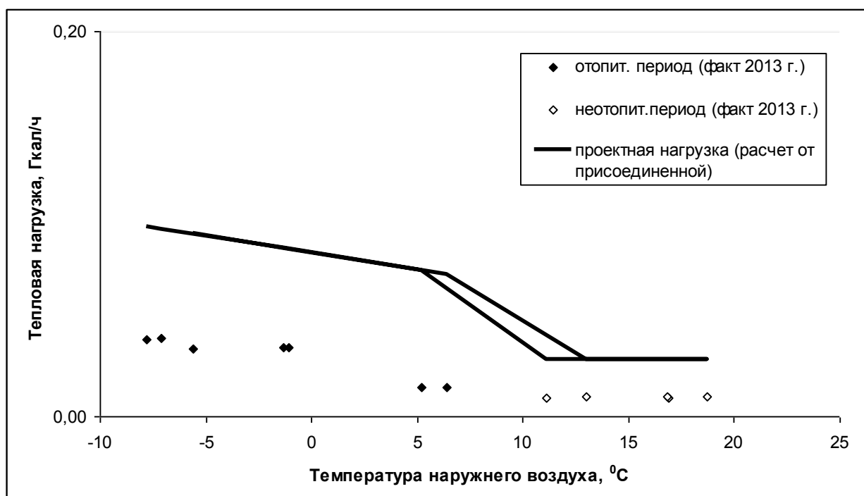
Рисунок 1.30. Зависимость тепловых нагрузок котельной д. Маврино ООО «ТеплоИнвест» от температуры наружного воздуха
