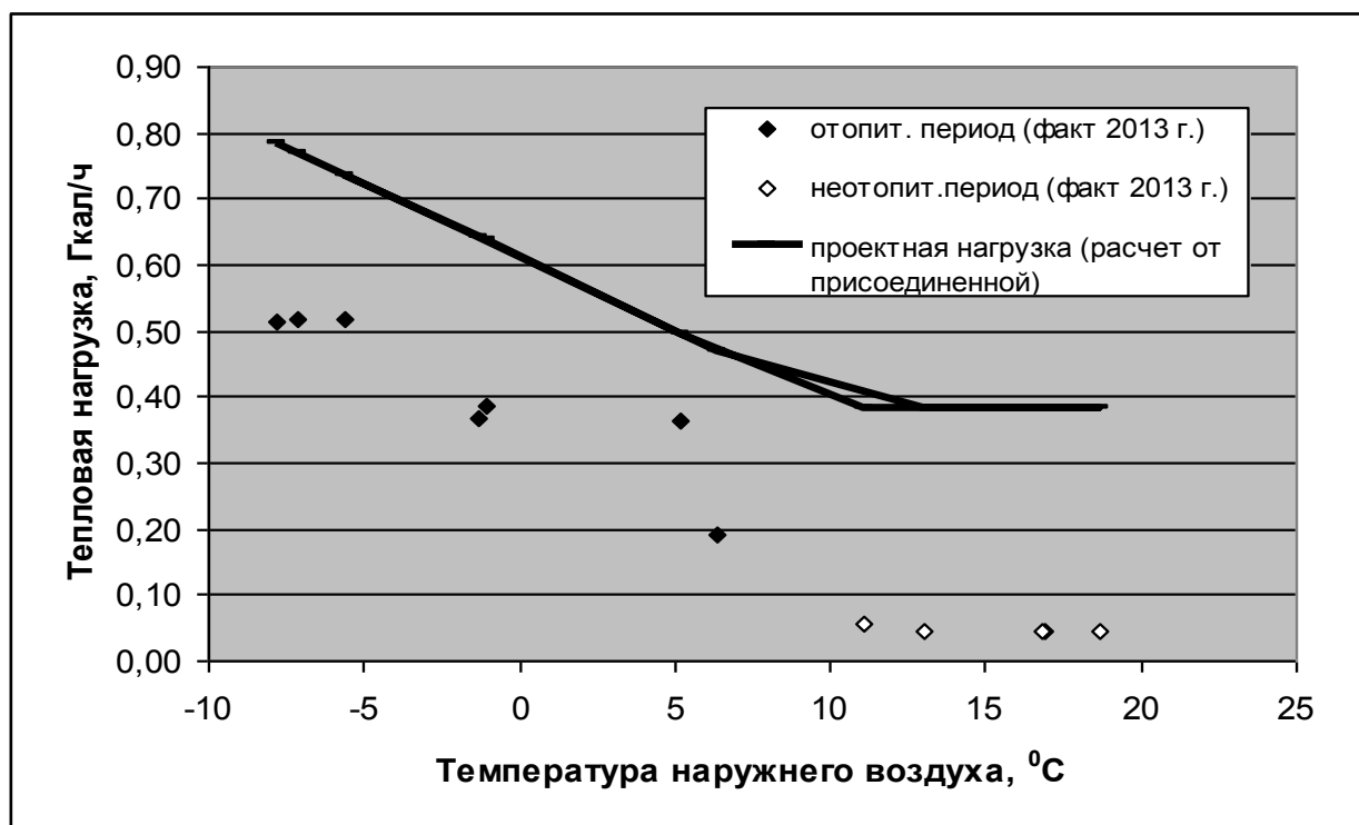
Рисунок 1.32. Зависимость тепловых нагрузок котельной п. Мещерский Бор ОАО «Водоканал МО» от температуры наружного воздуха
