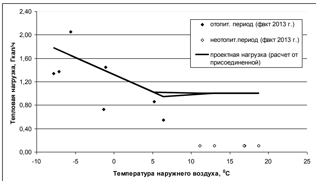
Рисунок 1.31. Зависимость тепловых нагрузок котельной п. Санатория «Белое Озеро» ОАО «Водоканал МО» от температуры наружного воздуха
